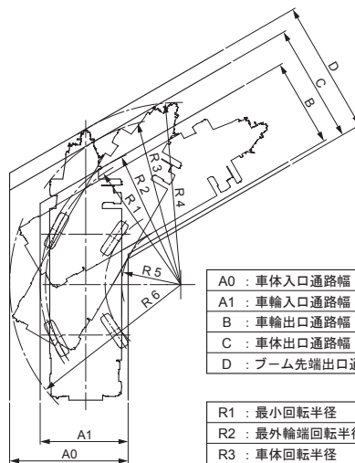
4輪ステアリングで右折する場合
